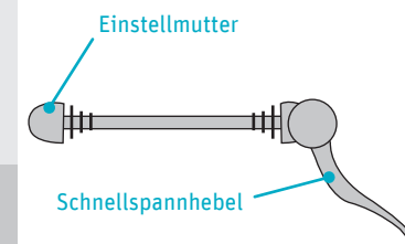
Schnellspannhebel geöffnet
